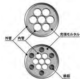
支柱断面図
