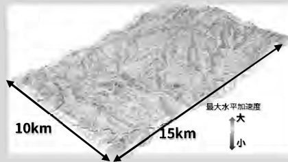
『FEMによる斜面の変位量解析』
